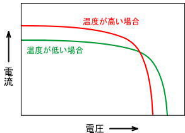
太陽電池の温度特性
