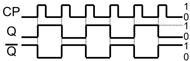
T-FF動作
